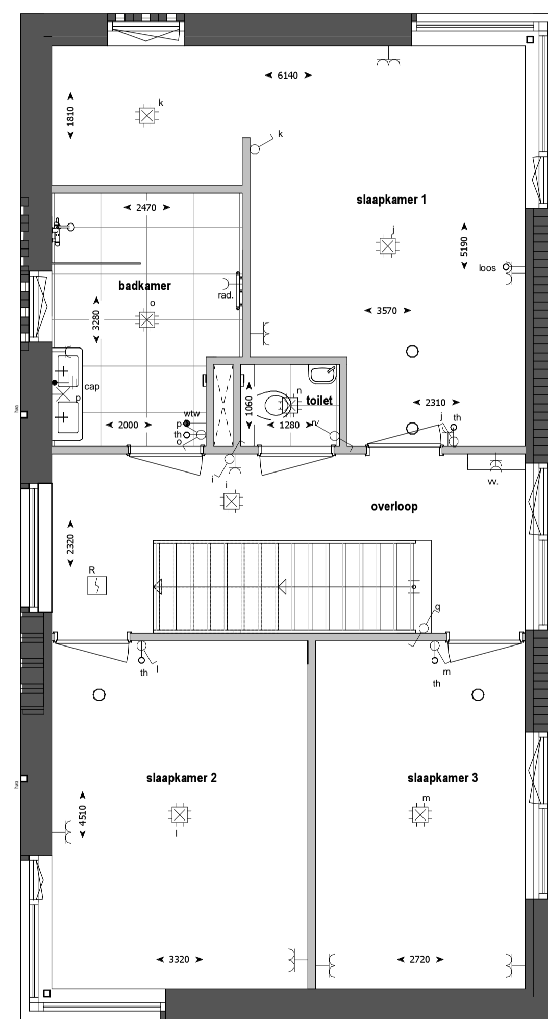
Eerste verdieping
