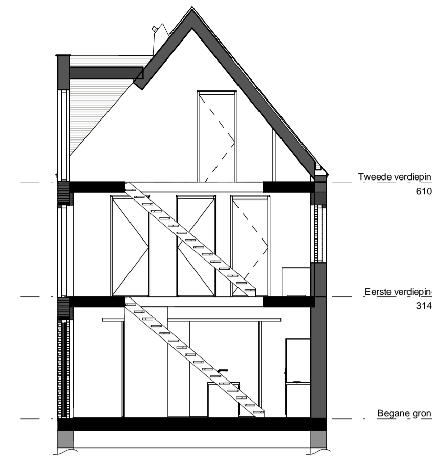
Doorsnede
